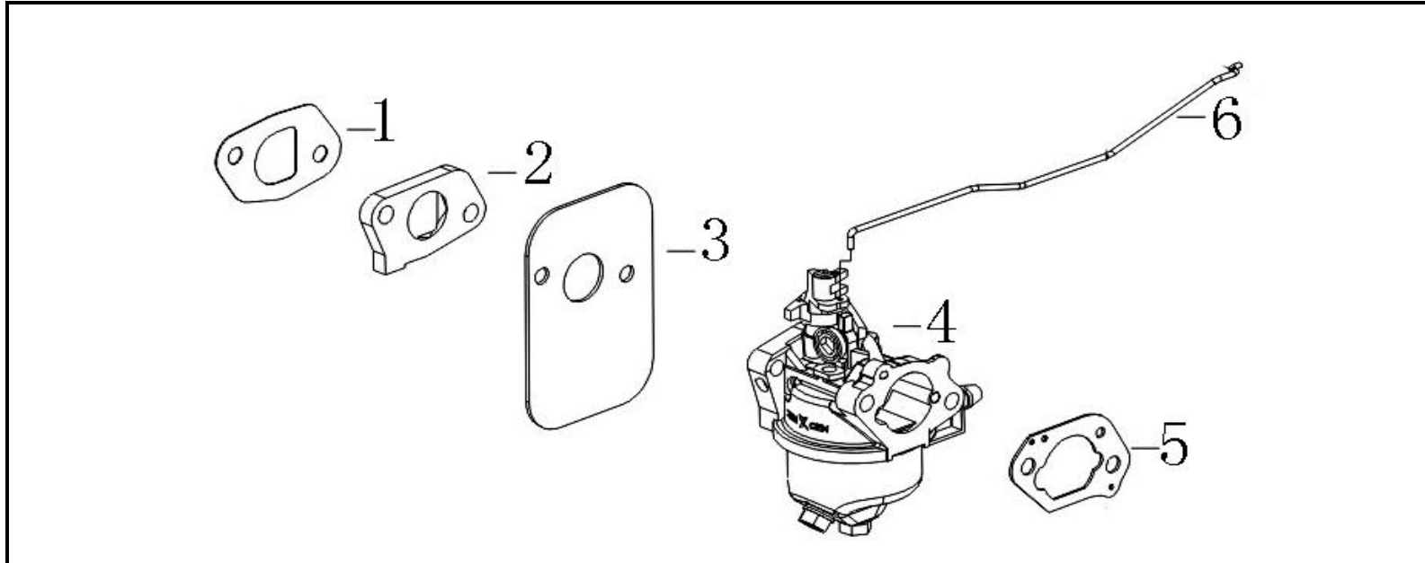
化油器 (CARBURETOR)
