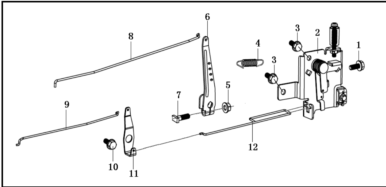
调速机构 (Governor)
