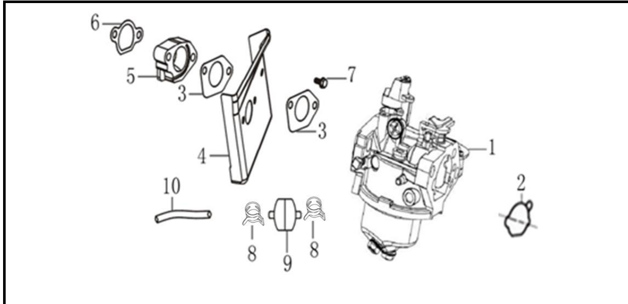
化油器 (Carburetor)
