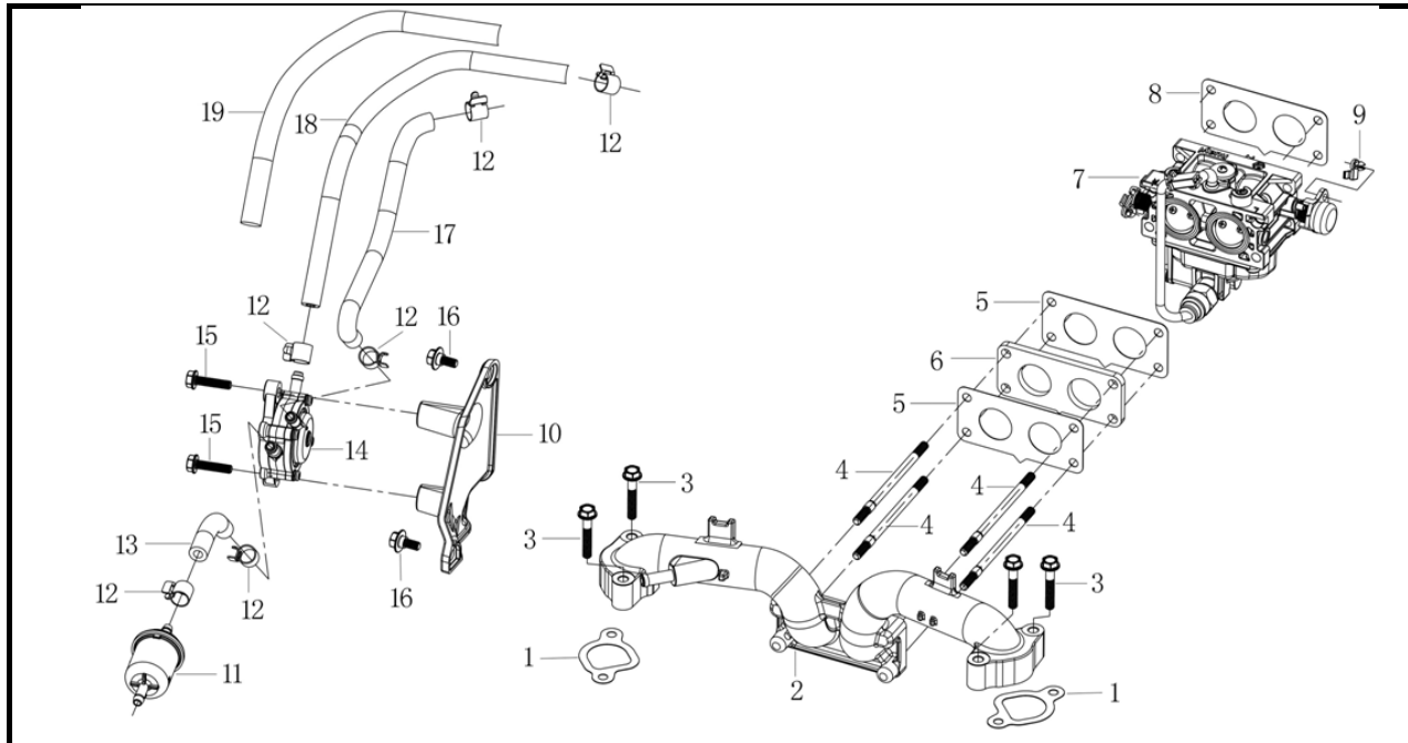
化油器 (CARBURETOR)
