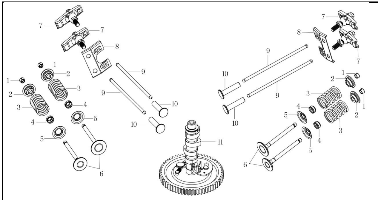
配气系统 (ROCKER,CAMSHAFT)
