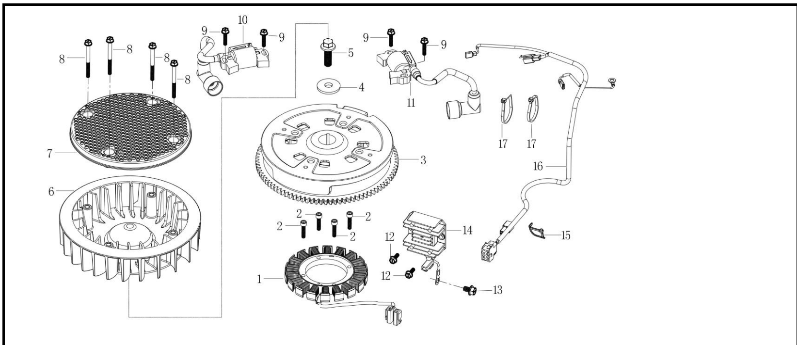
磁电机转子部分 (FLYWHEEL)
